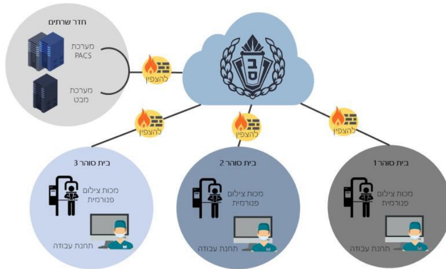
ציור 1 -תרשים תקשורת המערכות
